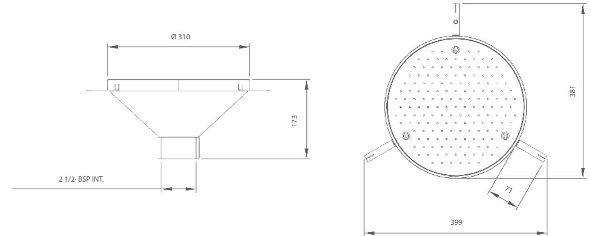
35078 REJA DE HIDROMASAJE DIÁMETRO 300 MM HORMIGÓN
