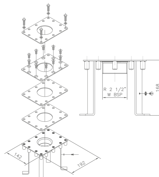
15833 ANCLAJE RECTANGULAR PISCINA PREFABRICADA
