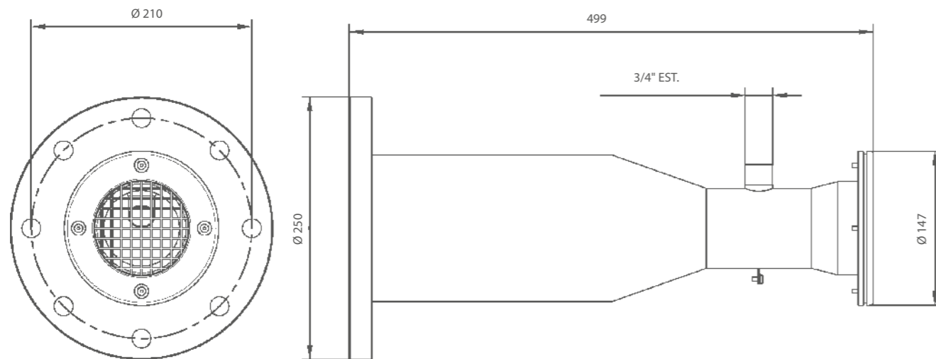
JET HIDROCANAL DINÁMICO HORMIGÓN
