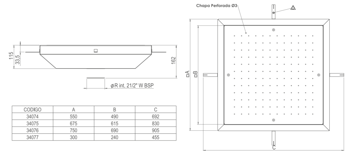
35076 REJA DE HIDROMASAJE 750 X 750 HORMIGÓN
