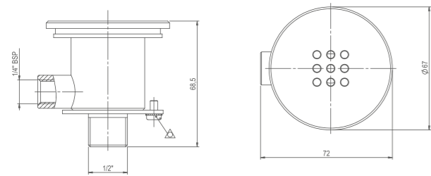
41282 CONJUNTO MINIJET CON EMBELLECEDOR DE 9 ORIFICIOS
