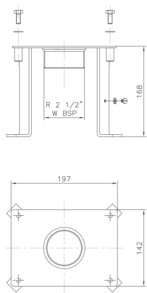
19983 ANCLAJE RECTANGULAR PISCINA HORMIGÓN
