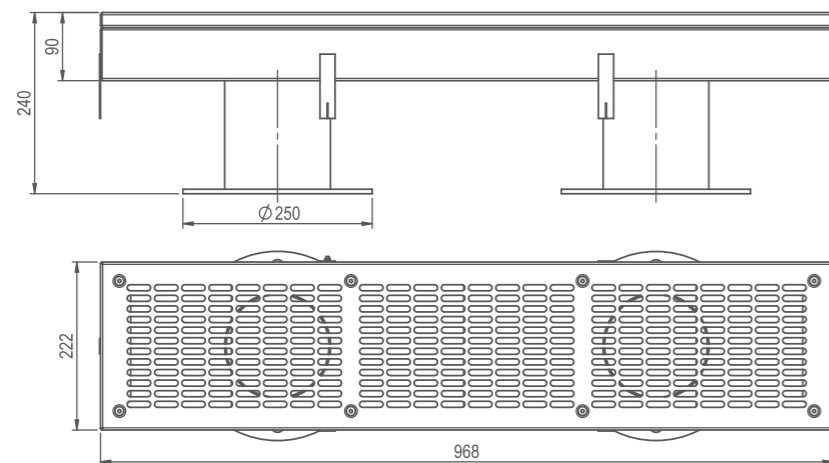
58814 CAJÓN ASPIRACIÓN GRAN CAUDAL 120 M 3 /H HORMIGÓN
